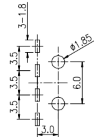
P.C.B LAYOUT
